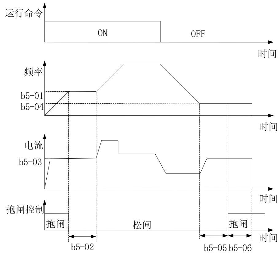
图5-31. 抱闸控制过程图
