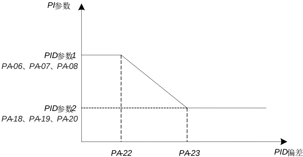
图5-24. PID参数切换
