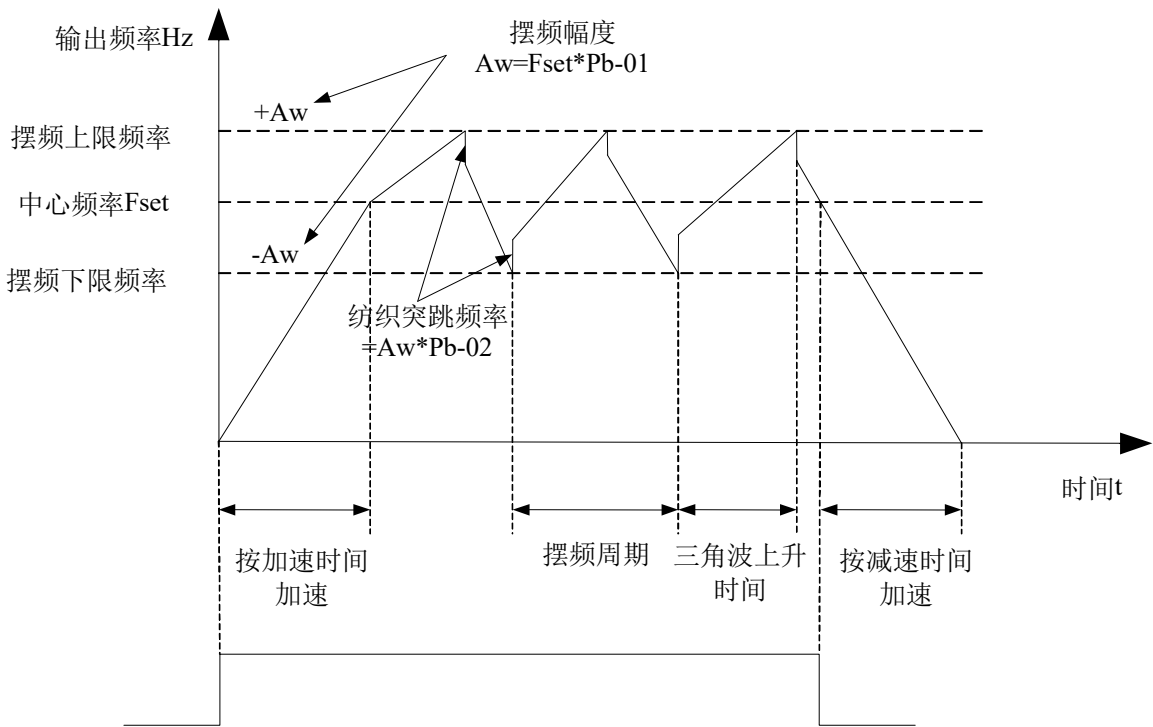
图5-26. 摆频工作示意图
