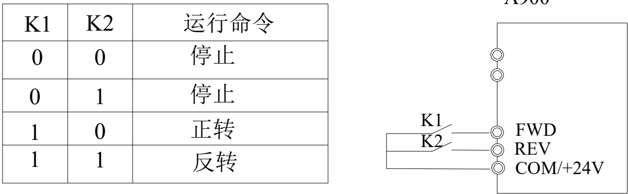
图5-8. 两线式运转模式2
