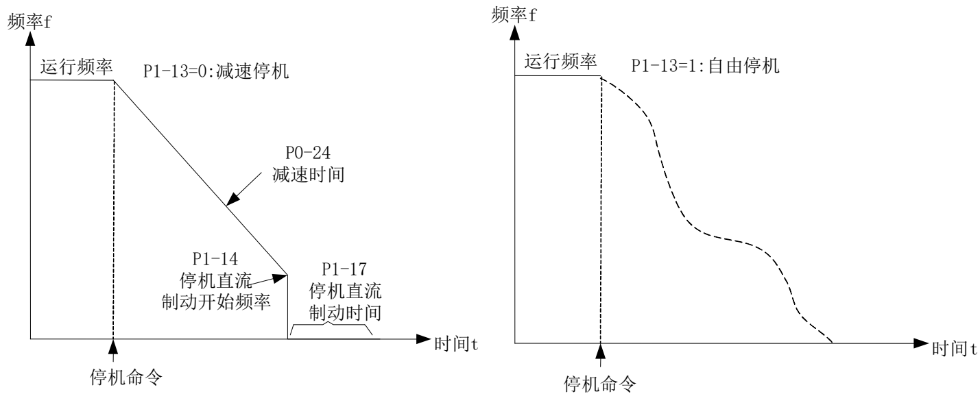
图4-13. 停机示意图
