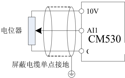
图 3-8.模拟量输入端子接线示意图
