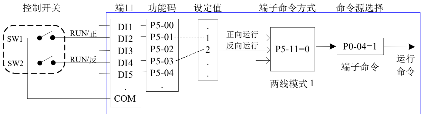
图4-8. 端子控制启停示意图
