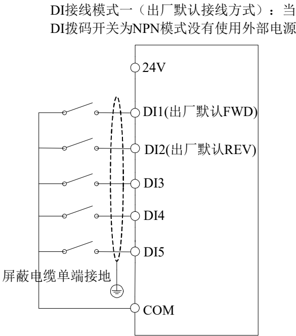
图3-9. 数字输入端子接线图
