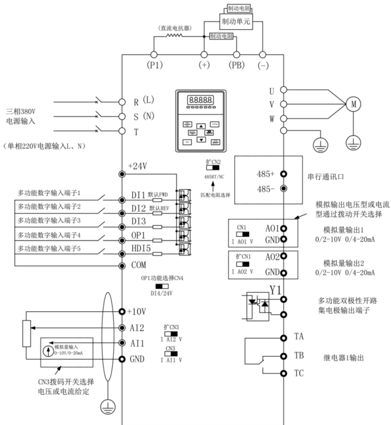
图 3-4 A900-30kw 及以上三相变频器基本接线示意图
