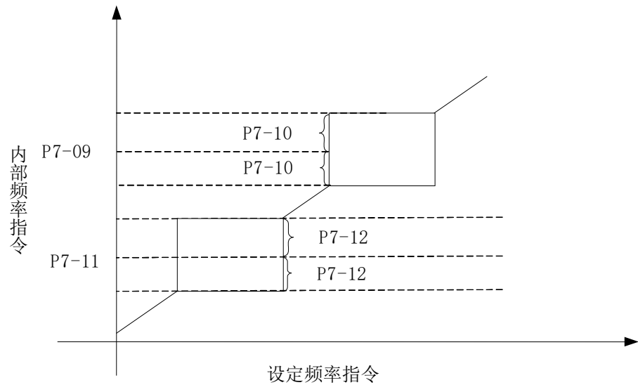
图 5-13. 跳跃频率示意图
