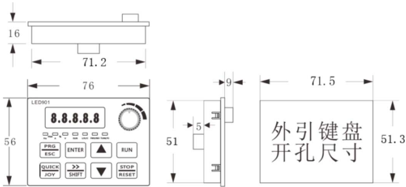
图 2-5.A901 LED 面板外形尺寸及外引开孔尺寸图
