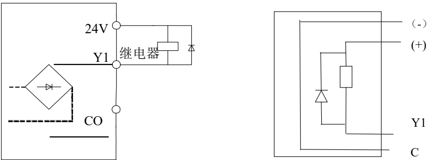
图3-10. 数字输出端子Y1接线示意图
