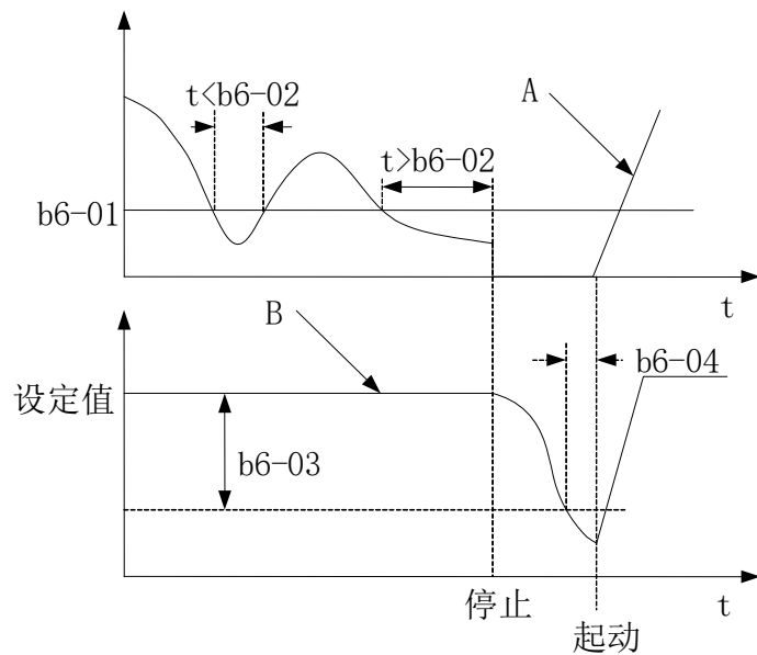
图5-32. 休眠过程频率图
