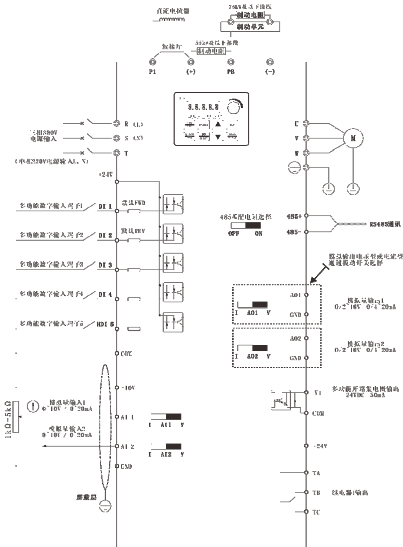
图 3-5. A900 变频器加 EX1 扩展卡接线示意
