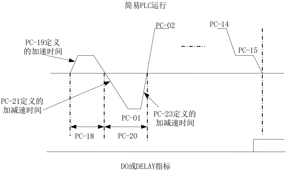
图5-29. 简易PLC示意图
