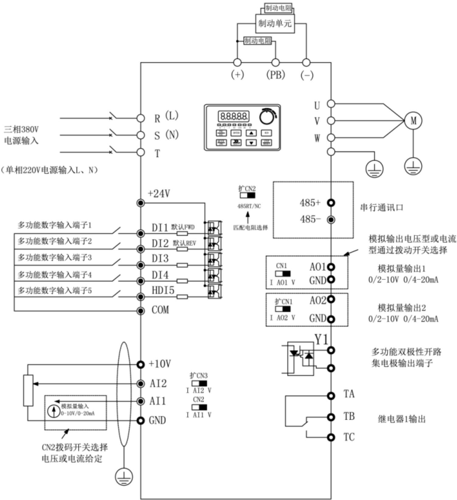
图 3-3. A900-22kw 及以下变频器基本接线示意图
