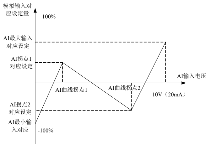
图5-30. 多点曲线对应示意图
