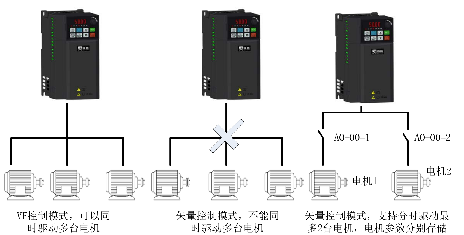
图 4-26. 多组电机的切换
