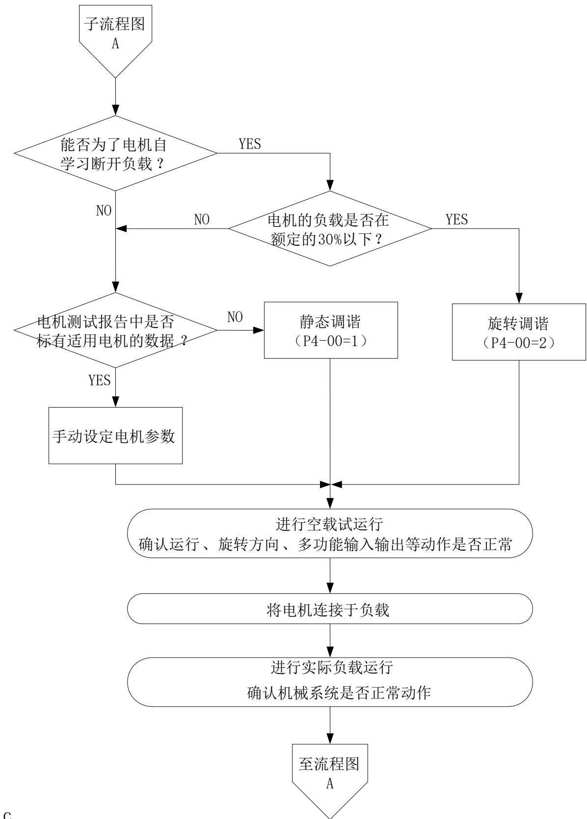
图 4-6. 开环矢量控制方式运行步骤
