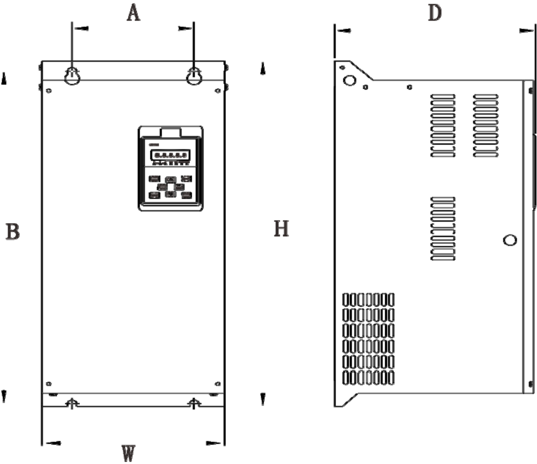
图 2-3.2.2kW 及以下塑胶外形尺寸及安装尺寸示意图
