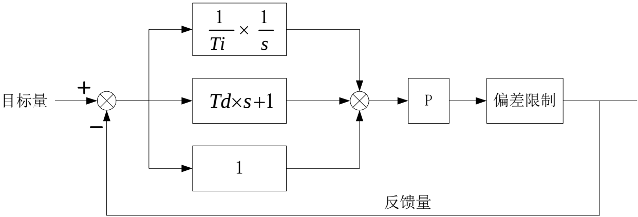
图5-23. 过程PID原理框图
