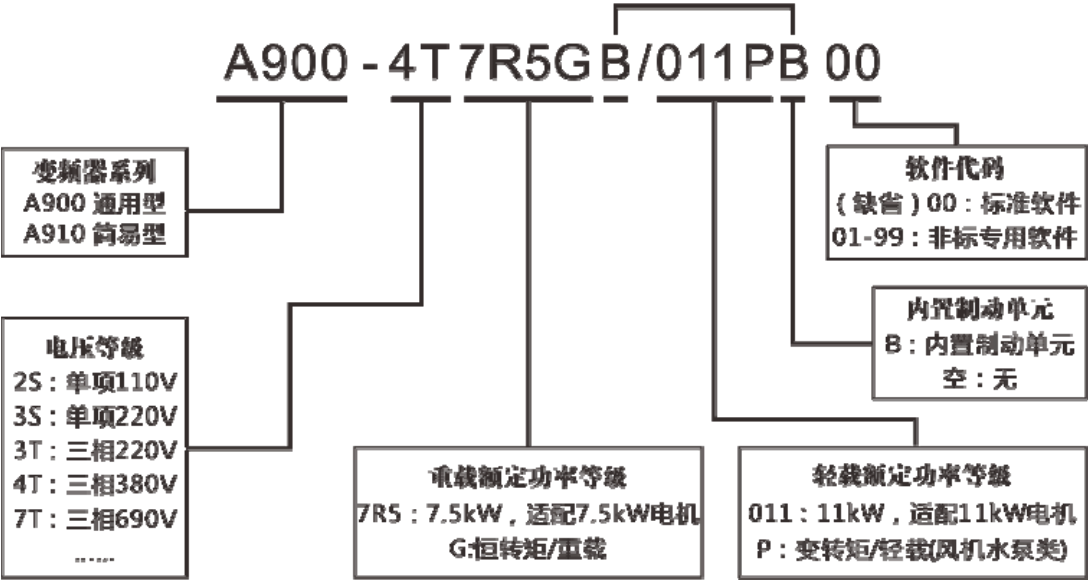
图2-1. 命名规格
