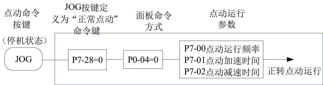
图4-15. 点动参数设定示意图
