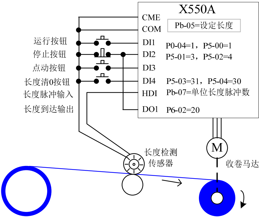
图 4-24. 定长控制功能常见应用举例
