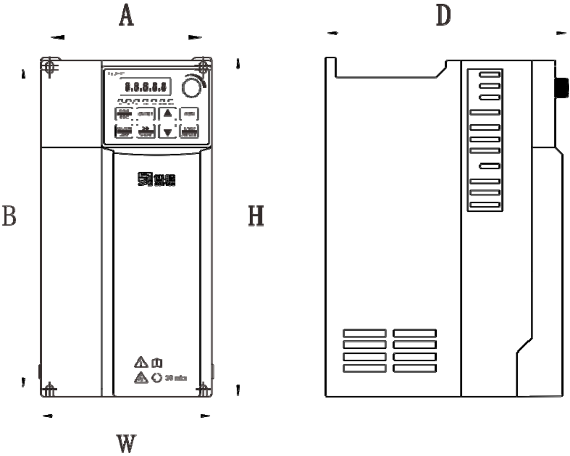
图 2-3.2.2kW 及以下塑胶外形尺寸及安装尺寸示意图
