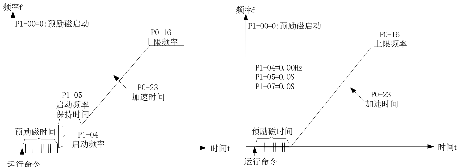
图4-12. 预励磁启动示意图
