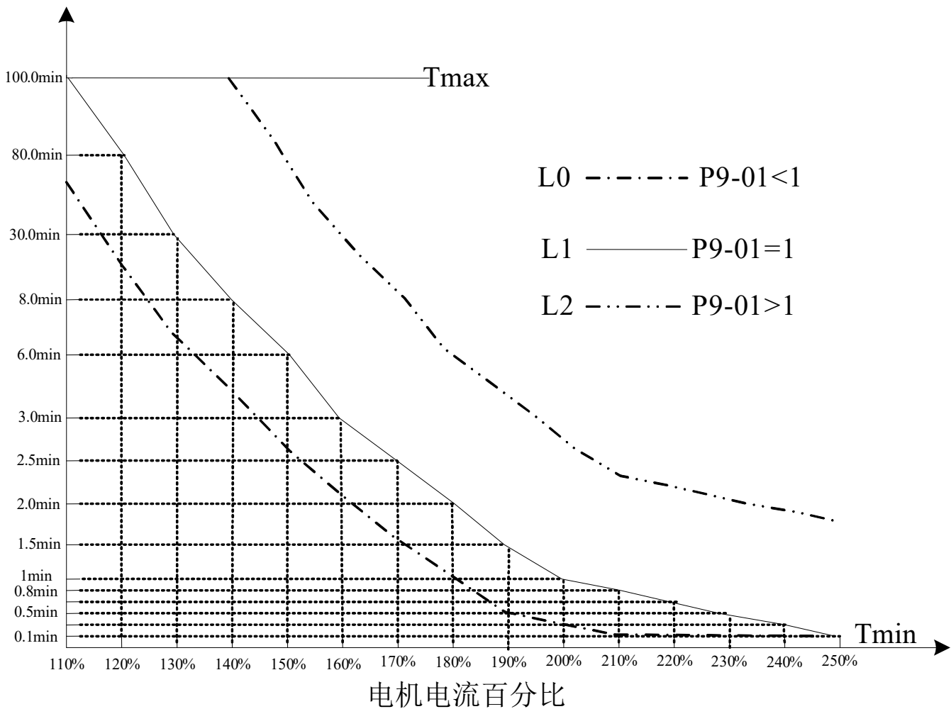
图5-21. 电机过载保护曲线
