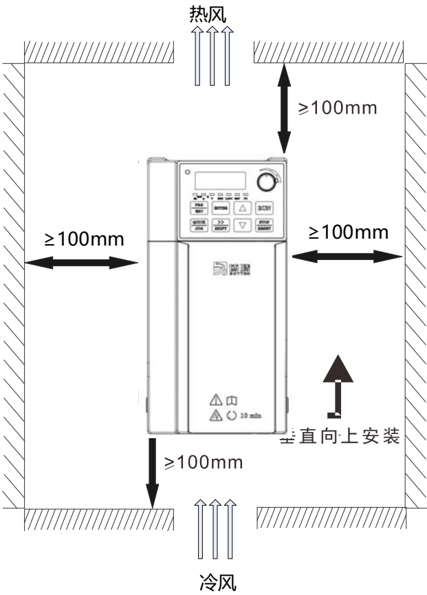
图3-1. 单体安装图
