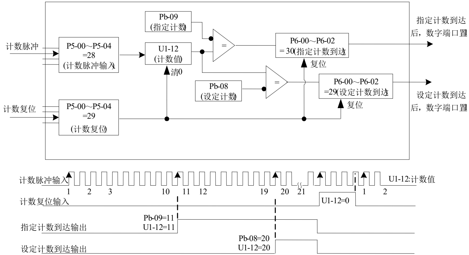
图 4-25. 计数模式功能码设置
