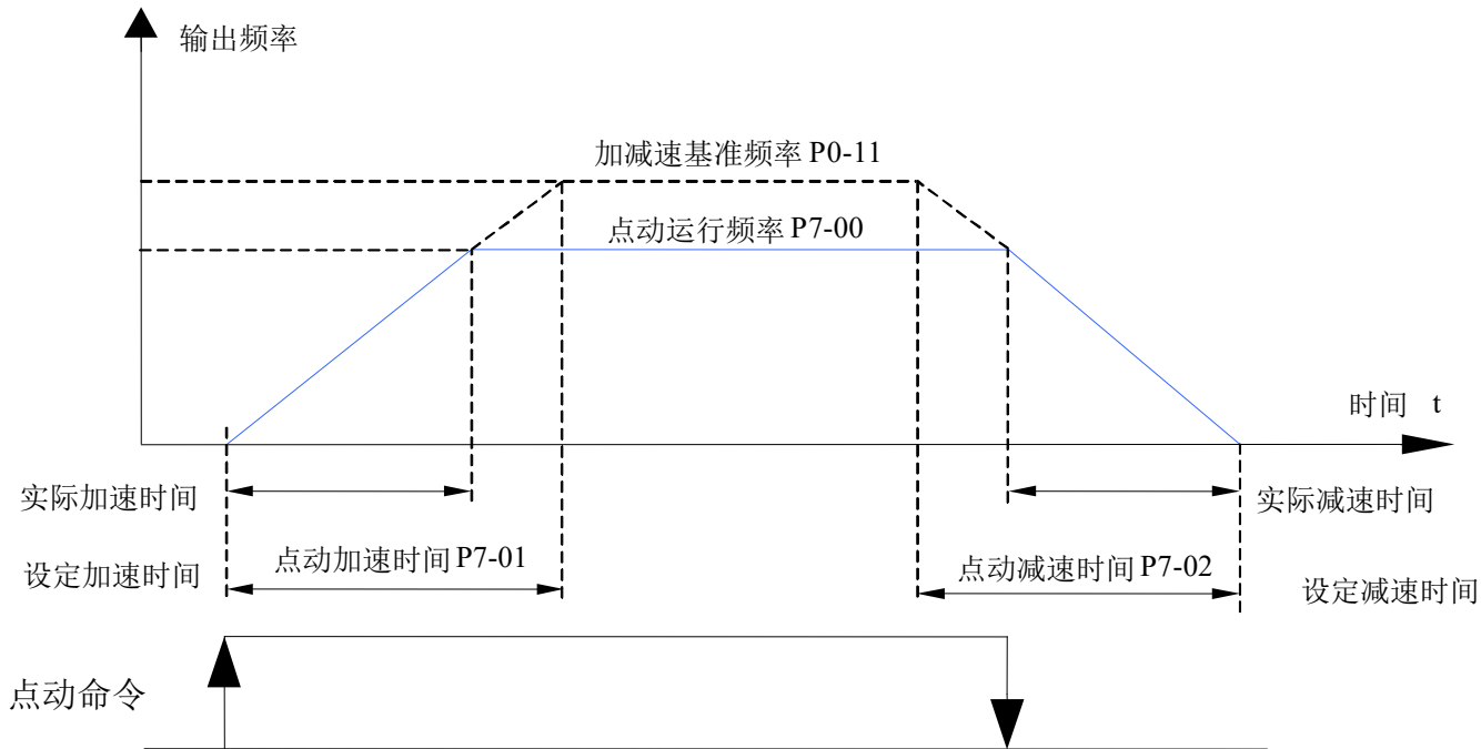
图4-14. 点动运行示意图
