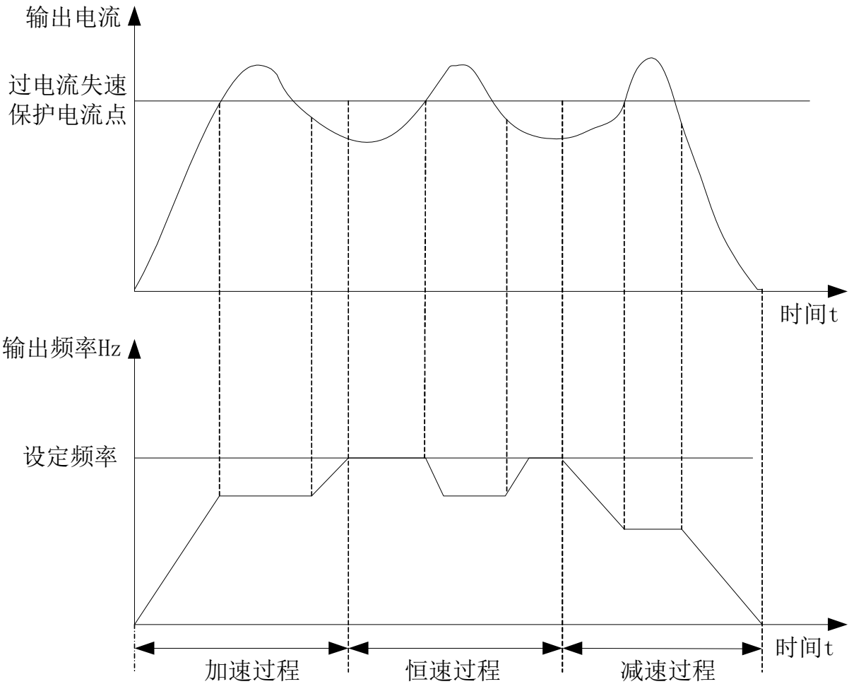
图5-22. 过流失速保护示意图
