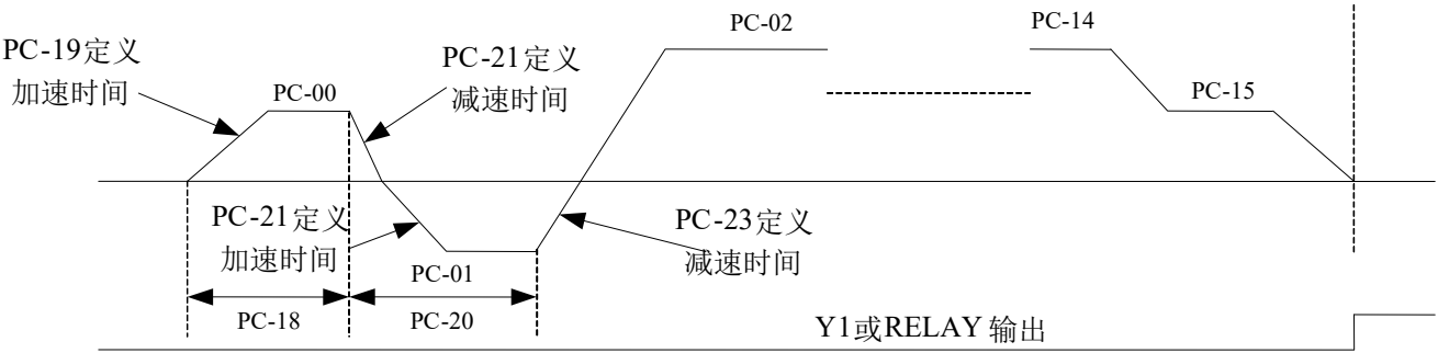
图 5-28. 简易 PLC 示意图
