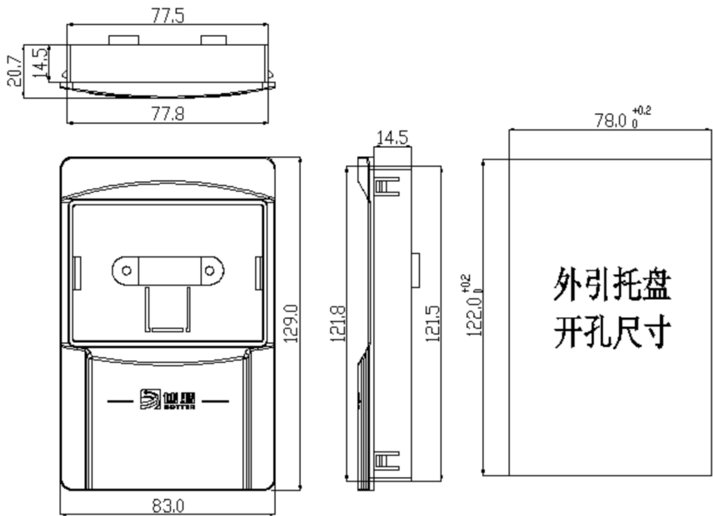
图2-6. A902 LED面板托盘外形尺寸及外引开孔尺寸图
