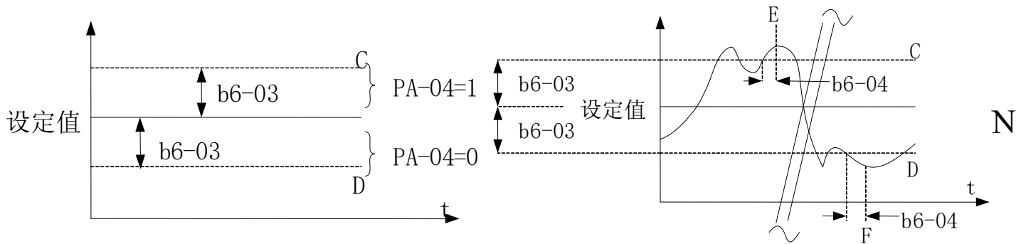
图5-33. 唤醒示意图
